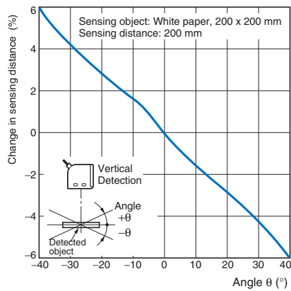
E3S-CL2 Vertical
