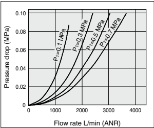
AF50-A Rc1
