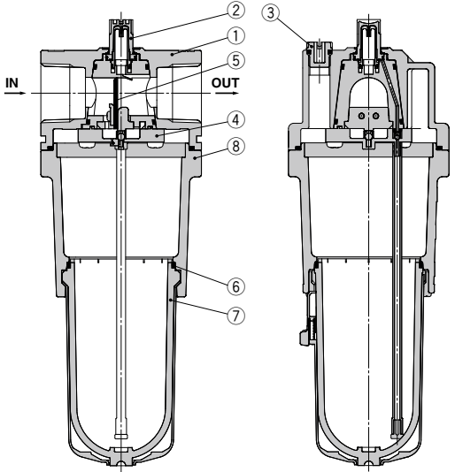
AL50-A/AL60-A
