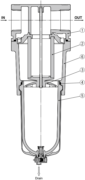
AF50-A/AF60-A
