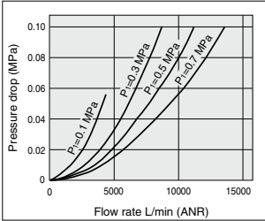
AF60-A Rc1
