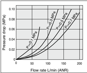
AF40-A Rc1/2
